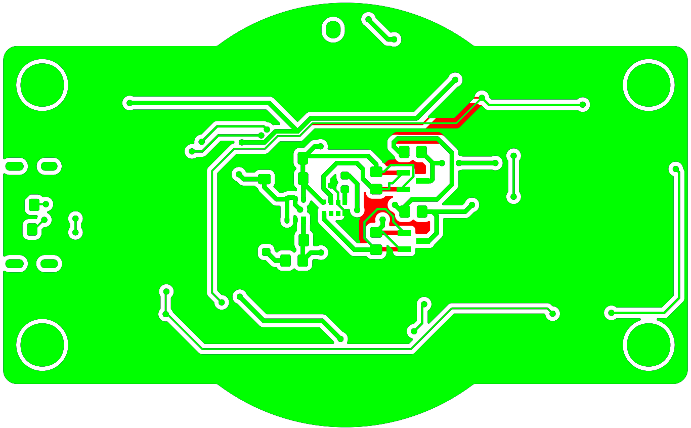
PCB_PAR_sensor-B_Cu.svg
