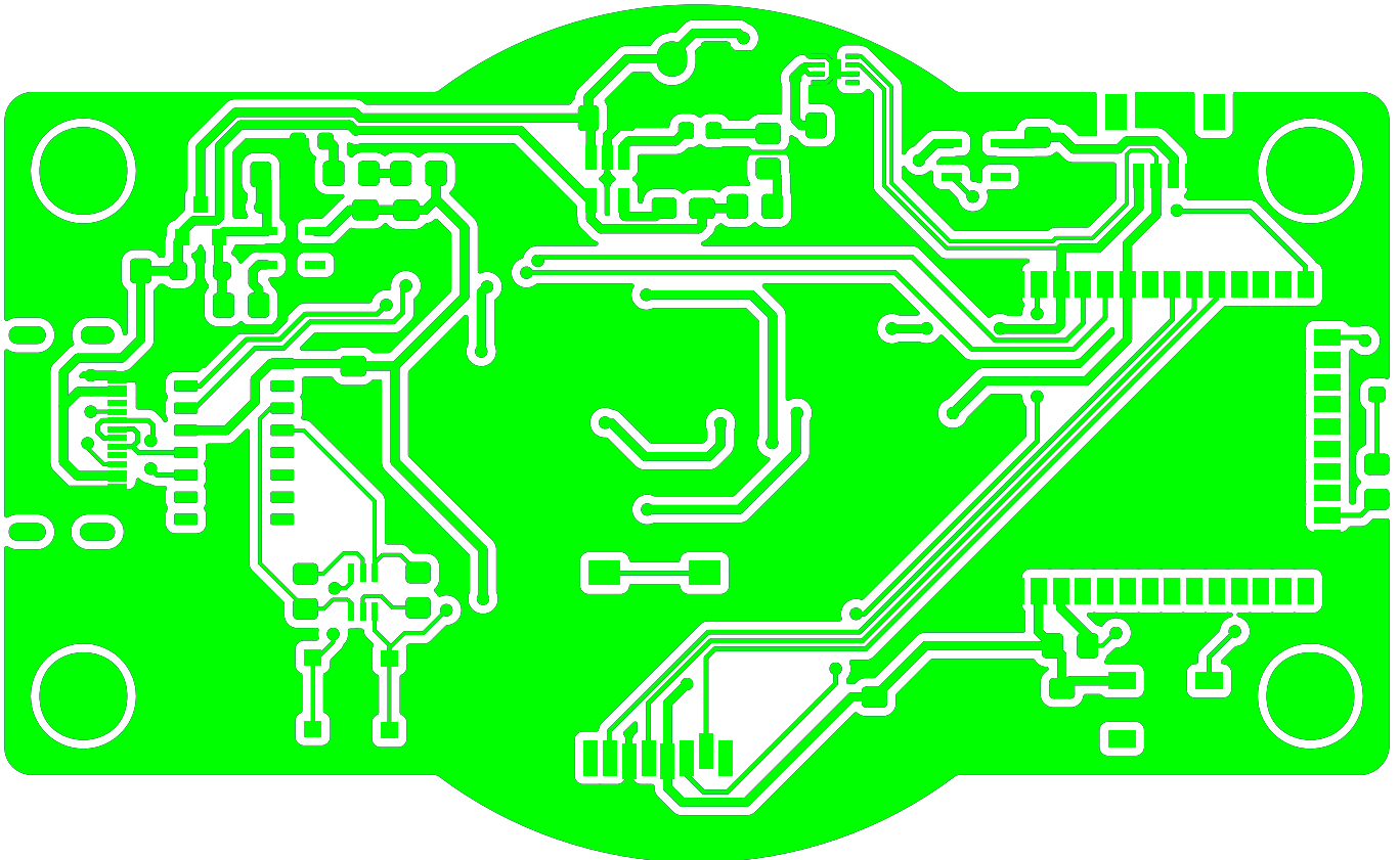
PCB_PAR_sensor-F_Cu.svg
